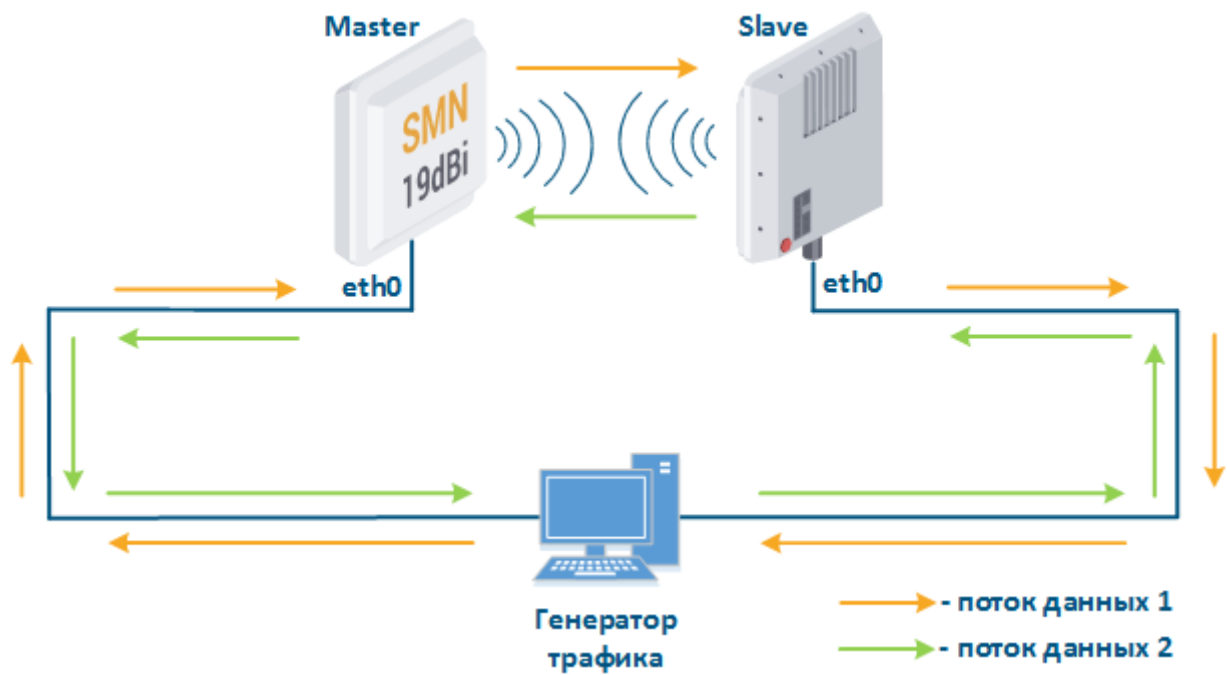
Рисунок 2 - Двухнаправленный тест пропускной способности
