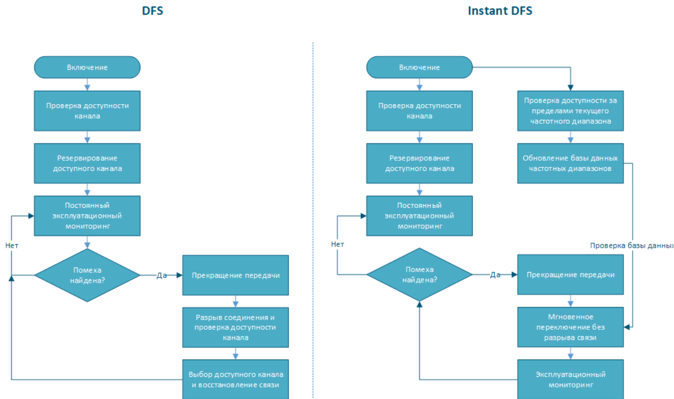
Рисунок - отличие DFS и Instant DFS
